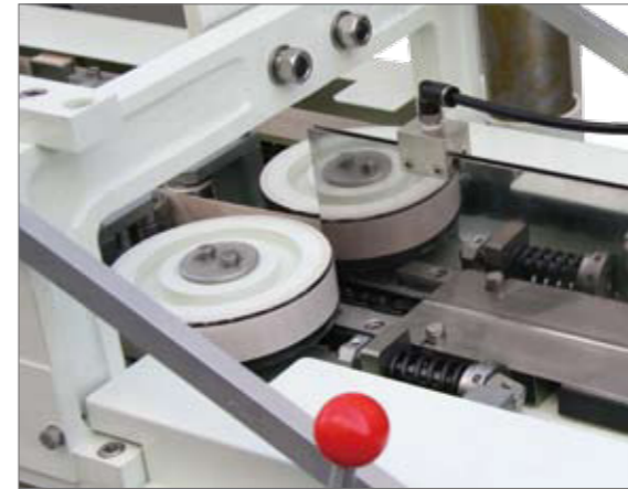
封口部分
